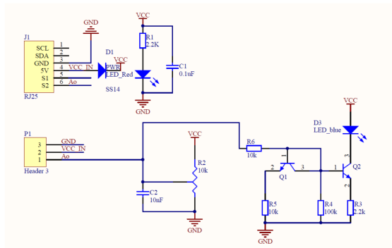
Figura 5: Documentación módulo electrónico MePotentiometer
